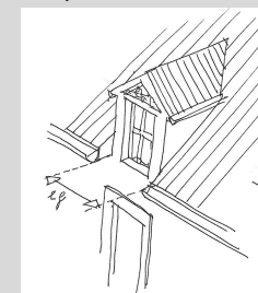
Fig. 51 : Lucarne de façade : \varphi \leq 2,20\text{m}
