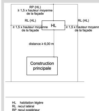
Fig. 55 : Reculs et distances en cas de HL
